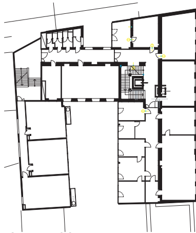
Grundriss OG
